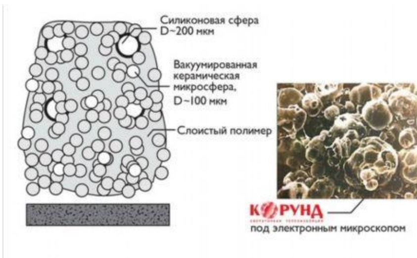
Рис. 1. Схематическое изображение теплозащитного покрытия КОРУНД.
