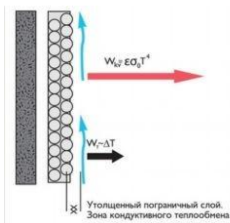
Рис. 6. Иллюстрация механизмов теплоотдачи от поверхности теплоизоляции КОРУНД
